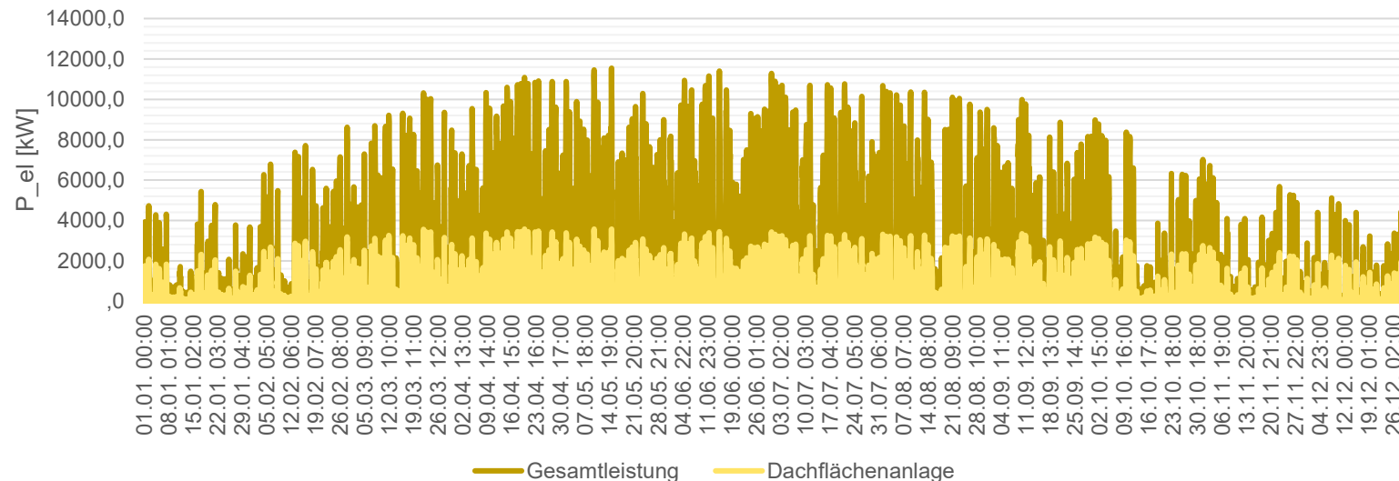
Leistung Photovoltaik-Anlage
